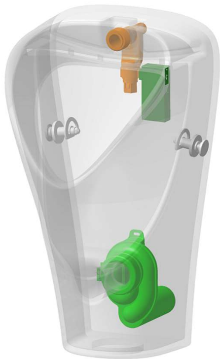
Ободковая керамика, Renova Trigonal (или другая) с настенным блоком
